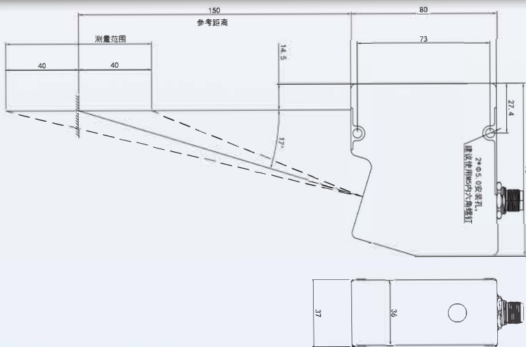
PL150R080W参数表
